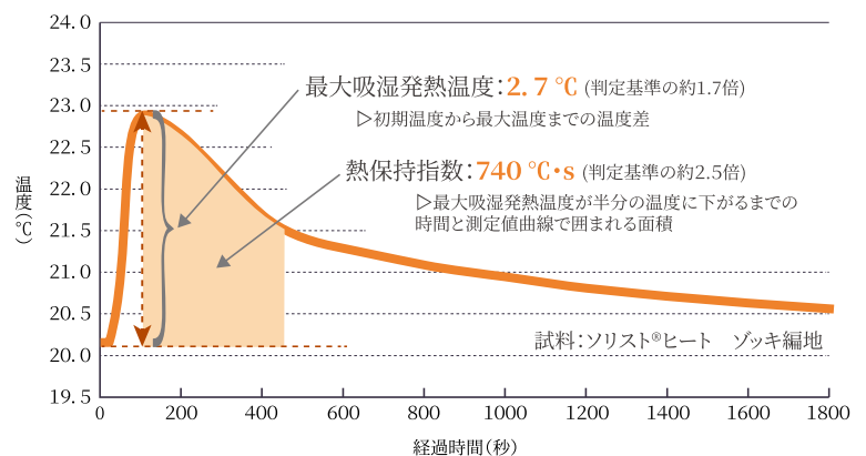
吸湿発熱性評価結果(JIS L 1952-1, 2)
